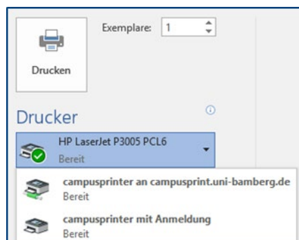
Abbildung 2: Drucker Auswahl 1
